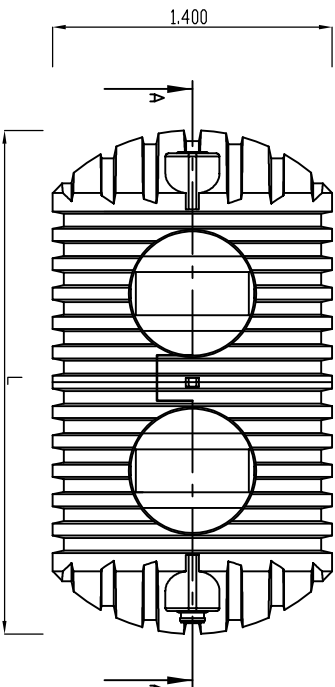
2-Kammeranlage aus Polyethylen mit zwei Domeinstiege DN600
