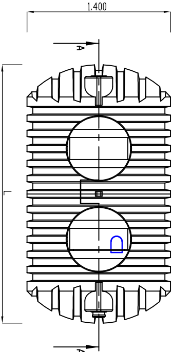
3-Kammeranlage aus Polyethylen mit zwei Domeinstiege DN600
