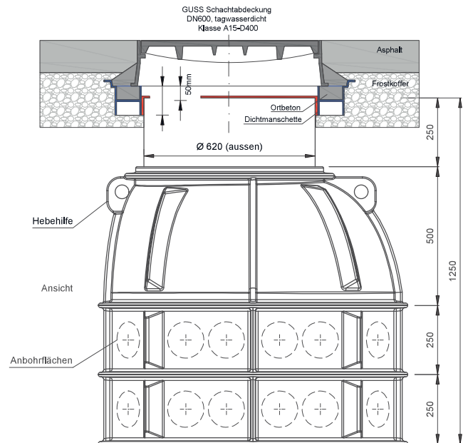
Beispiel: Tagwasserdichte Abdeckungsvariante
