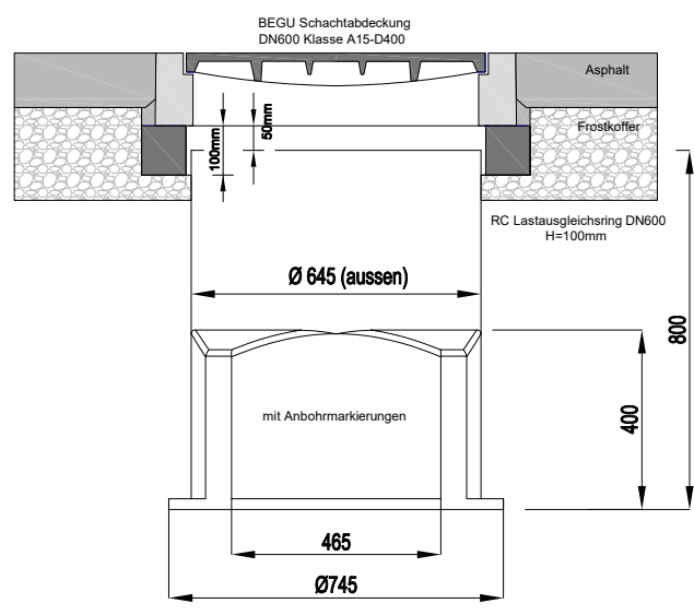
Beispiel: Sanddichte Abdeckungsvariante
